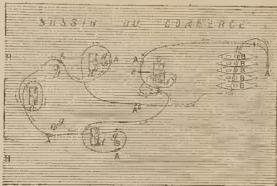
Fig. 3. - Trazado del camino recorrido por el Goubet durante las pruebas públicas de 13 de abril de 1890 en Cherburgo. - A, El Goubet estacionado delante de los cinco torpederos B. - G, Balsa inmovilizada por medio de áncoras - H, Boyas de amarradero. - e, Percha móvil. - f, Hélice. - g, Pequeñas boyas. - HII, Puercas de comunicación de la concha con el mar abiertas. - AAAA, El Goubet á diversas profundidades. - La línea de puntos doble indica el paso por debajo de los cinco torpederos y de la balsa.
